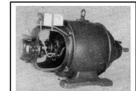
Die häufigste Form des Störschutzes: Der Doppelblock mit Erdung am Gehäuse (einer Gleichstrommaschine).
