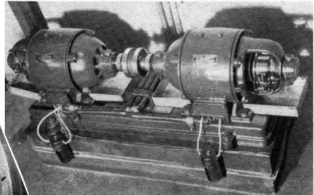
Links: Abb. 6. Ein Spezialkon- densator für Drehstrom- maschinen.
