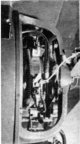
Abb. 4. Diese praktische An- klemmvorrichtung vereinfacht die Montage des Stör-schutz kondensators auf wenige Handgriffe.
