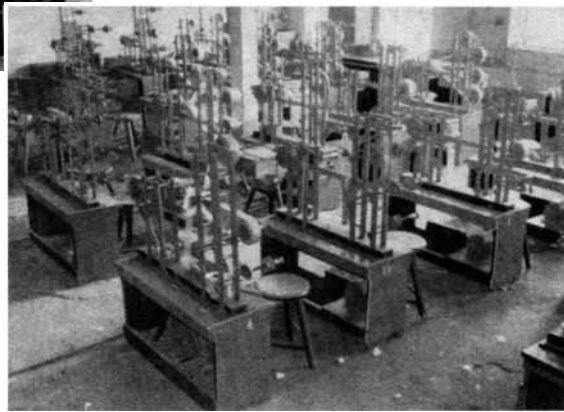
Unsere Bilder zeigen Ausschnitte aus der Fabrikation von Störschutzkondensatoren in den Betrieben der Fa. L. Flörshcim, München. Wir sehen die Wickelei, die Stapel der gepreßten Kondensatoren, fertig zum Einhängen in das Paraffinbad und ganz oben einen Vielfachblock mit den zahlreichen Kondensator-Wickeln im Innern u. der verwickelten Schaltung.
